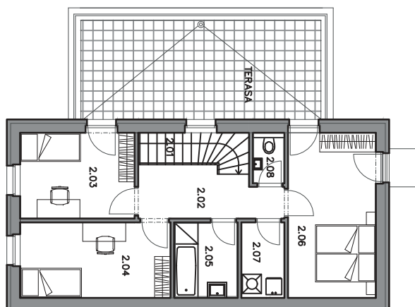
PŮDORYS 2.N.P.
