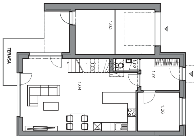
PŮDORYS 1.N.P.
